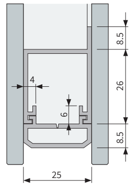
Section D-D
